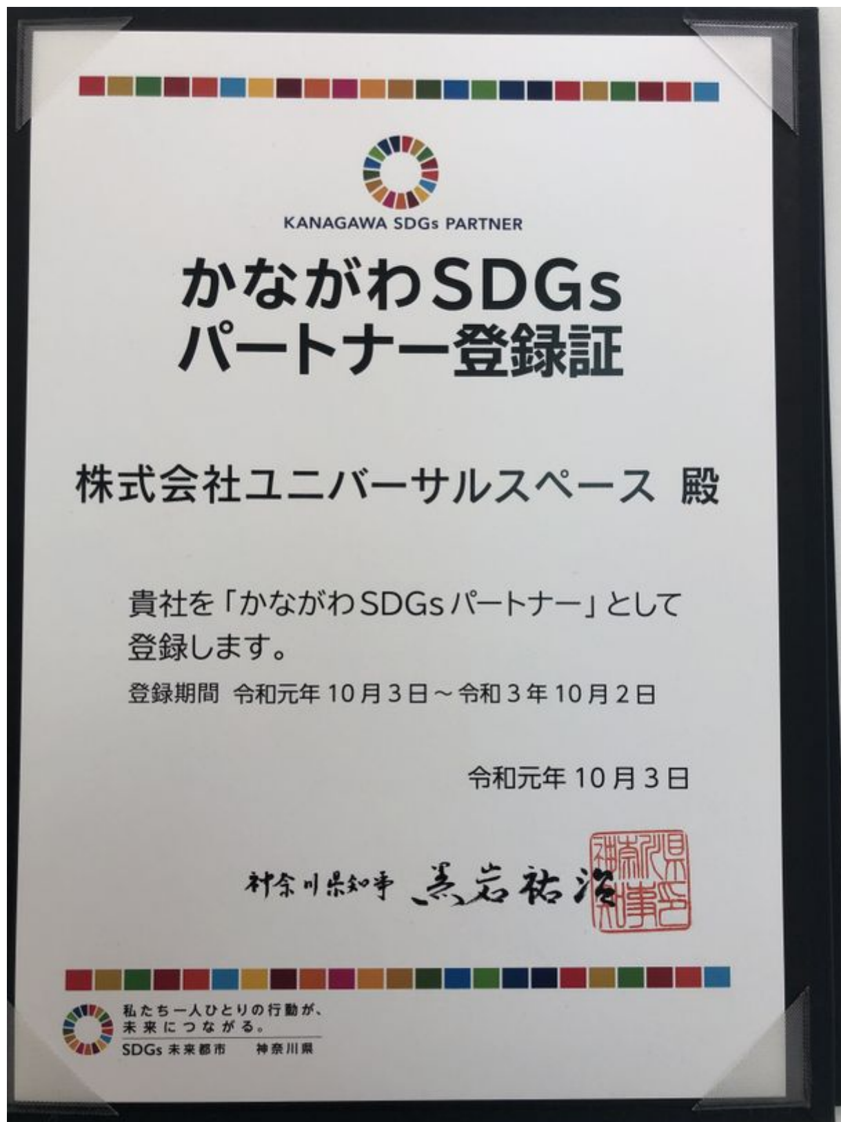
登録証
